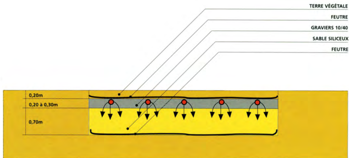
COUPE TRANSVERSALE
