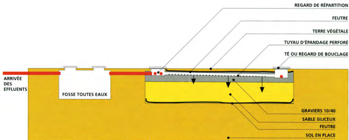
COUPE LONGITUDINALE
